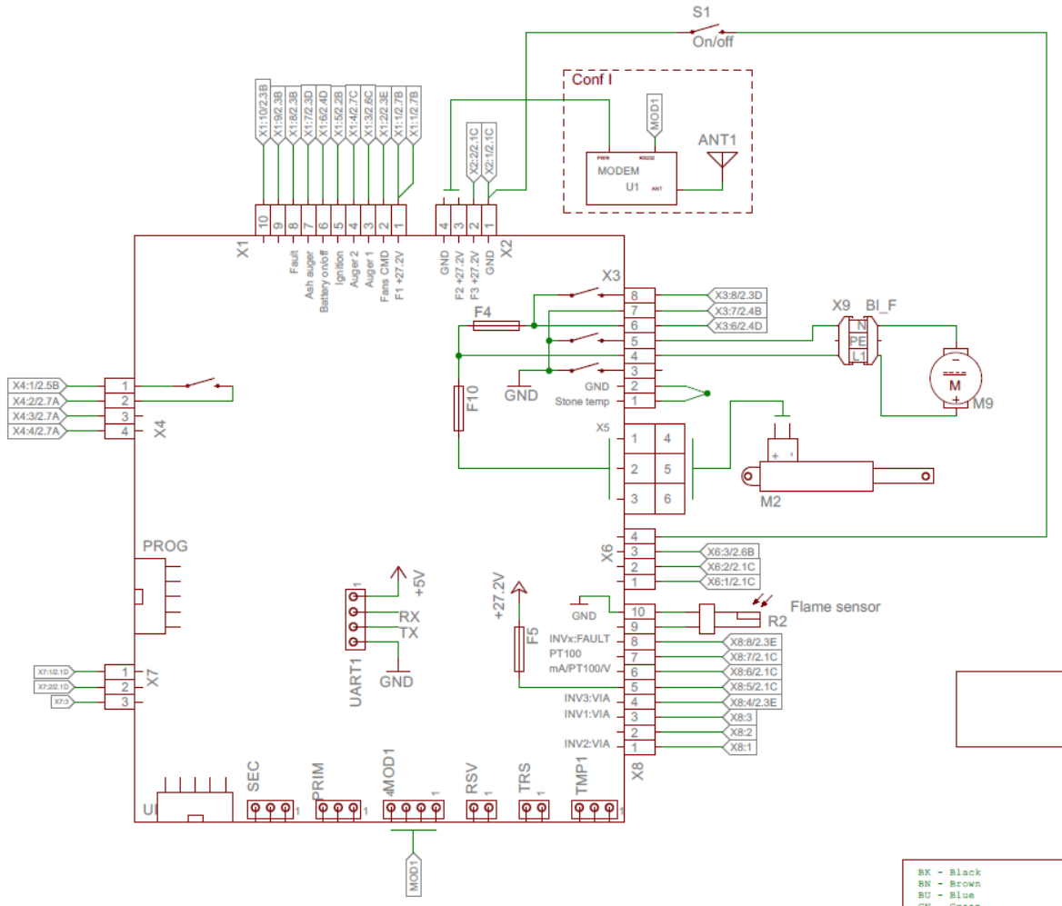
Figur 20 El schema
