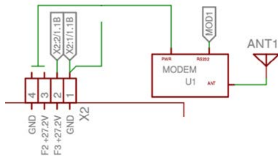
Figur 12 Anslutning av modem
