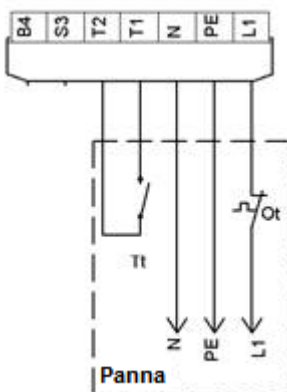
Figur 10 X11 anslutningar
